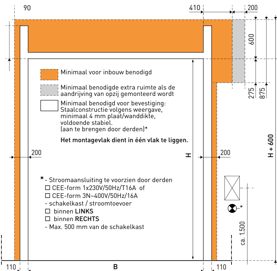
[ Vooraanzicht ]
