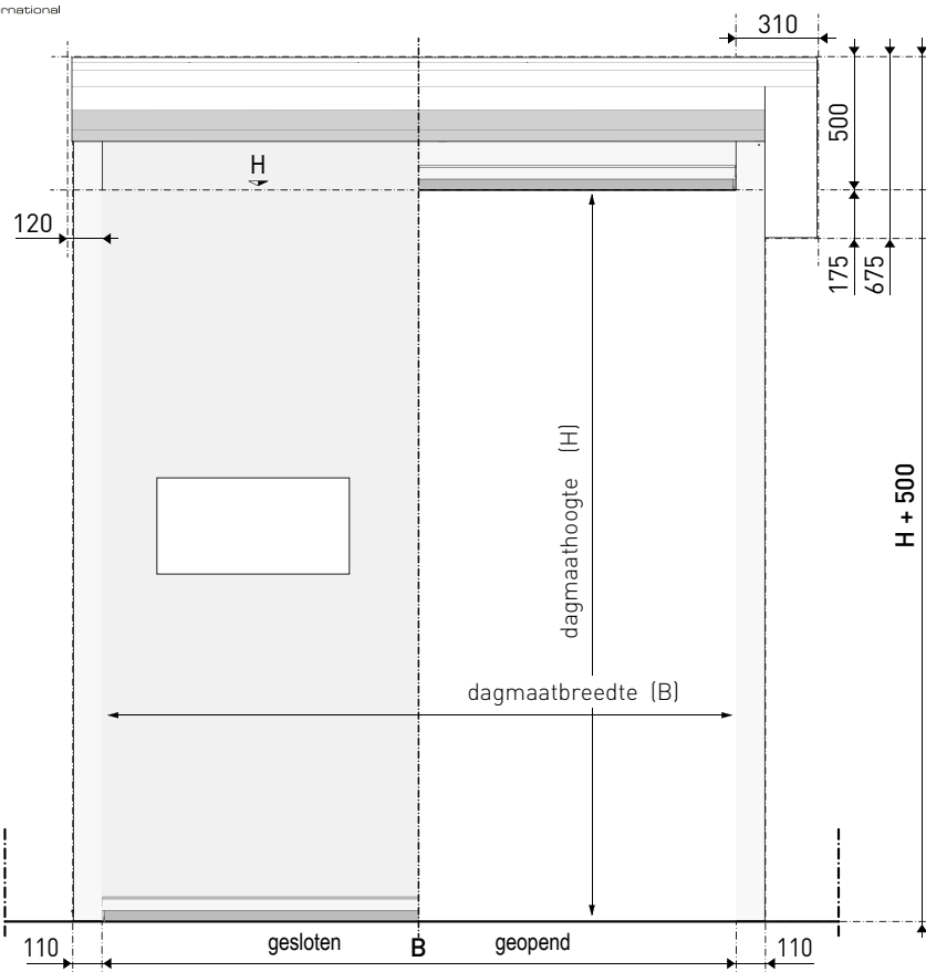
[ Vooraanzicht ]
